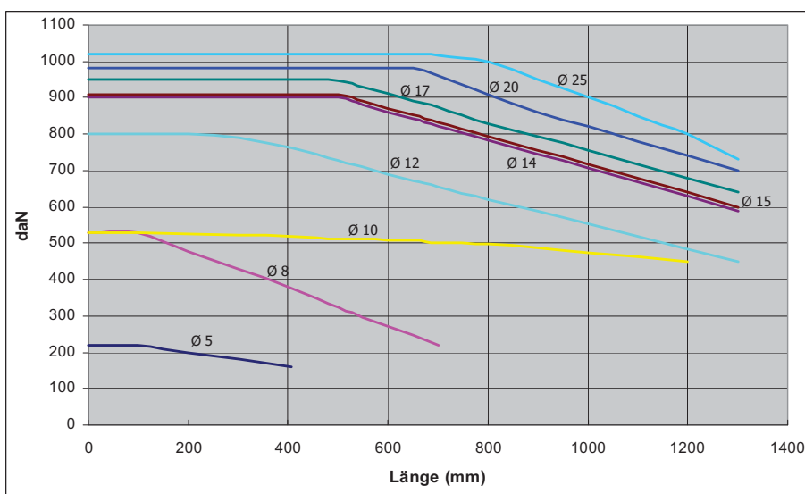
statische Belastung Achse, feste Einspannung (IGM, M, AGM)
