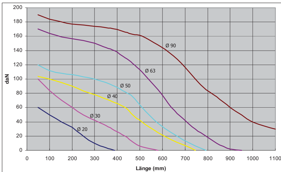
statische Flächenbelastung Kunststoffrohr
