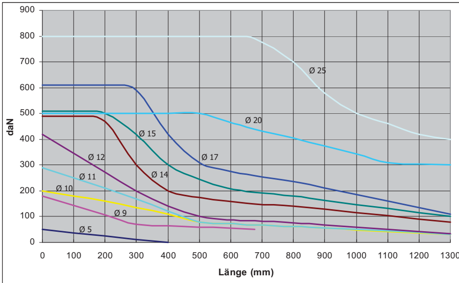
statische Belastung Achse, lose Einspannung GL, FA, SW
