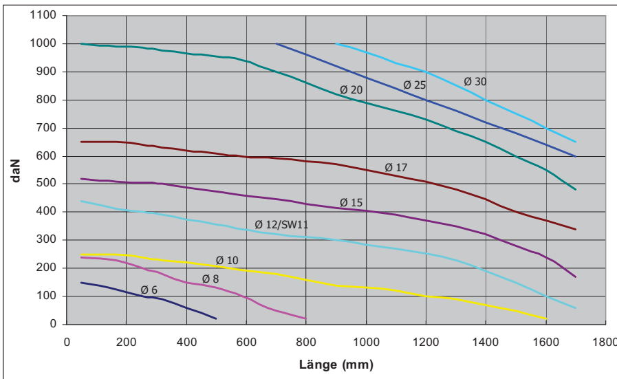
Belastung Achse, fest eingespannt
