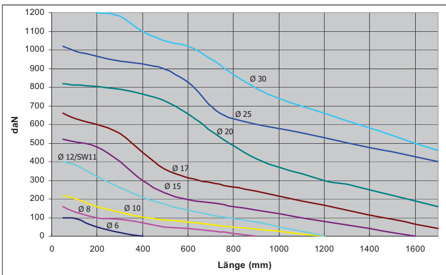
Belastung Achse, lose eingelegt
