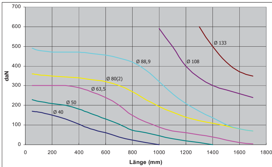
statische Flächenbelastung Stahlrohr
